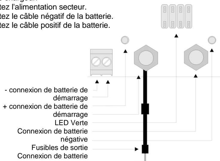
Illustration 3. Emplacement des connexions de la batterie
