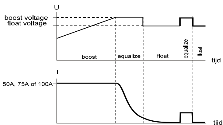
Illustration 1. La caractéristique de charge IUoUo
