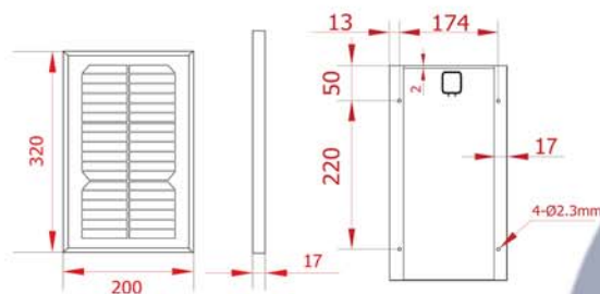
DIMENSIONES/DIMENSIONS ESF-5MA ESF-5PA
